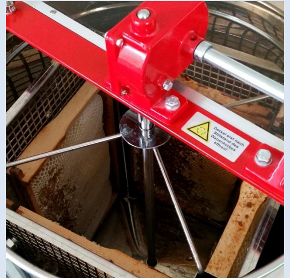
Beim Schleudern bewirken die Fliehkräfte, dass der Honig aus den Waben fließt
